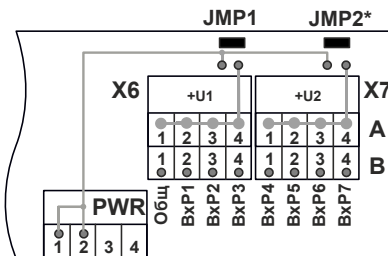
Рис. 4.5 – Организация питания датчиков давления
